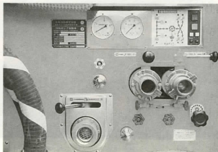
消防車のポンプ操作パネル
