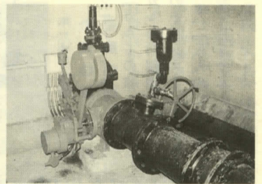
配水池の緊急遮断弁
