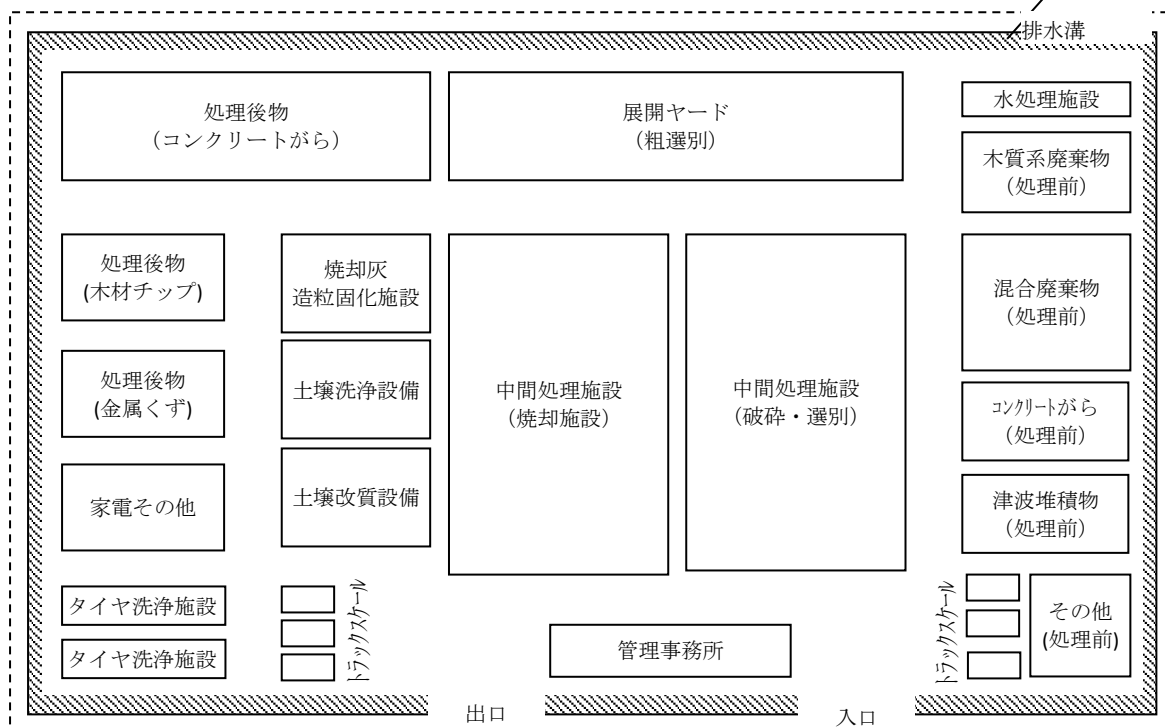
図3-8 二次仮置場レイアウト
